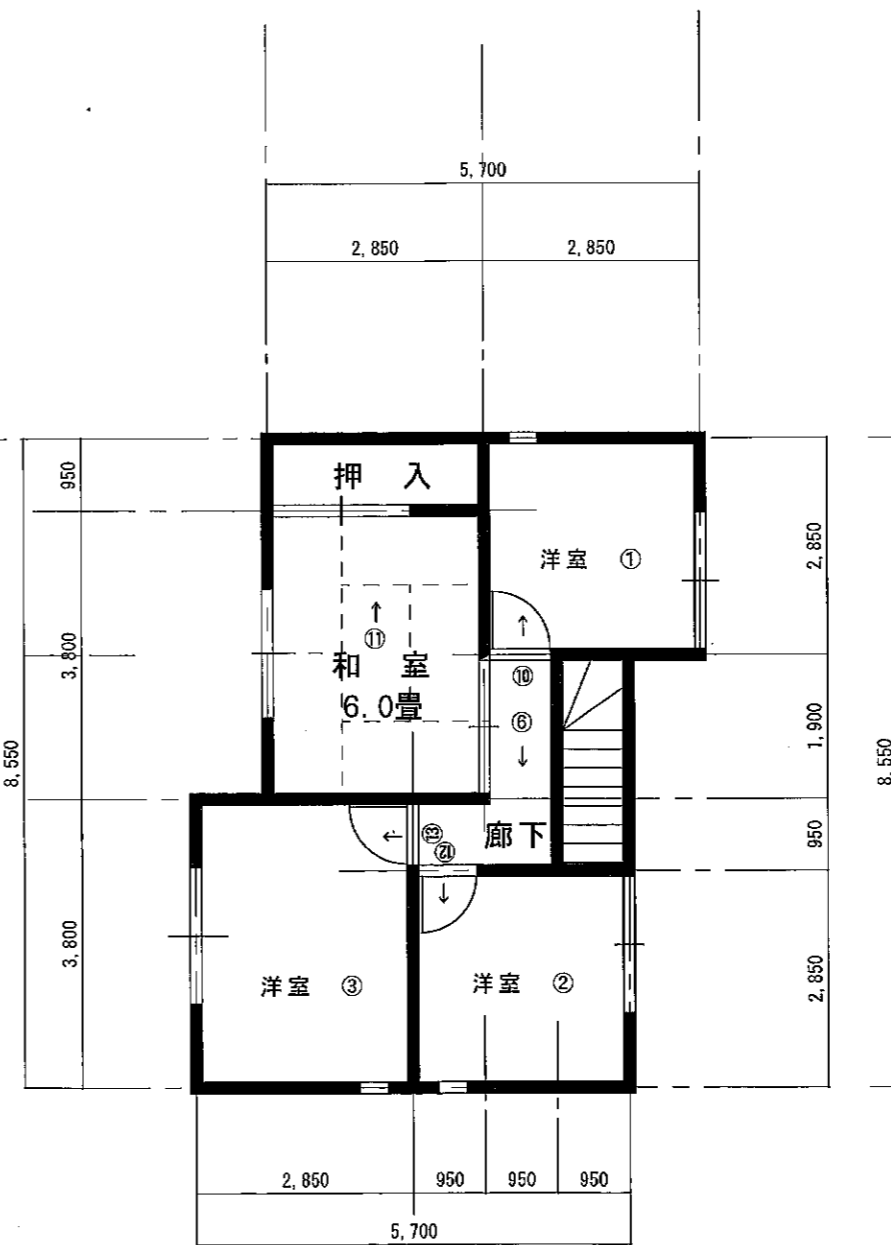
2階平面図
