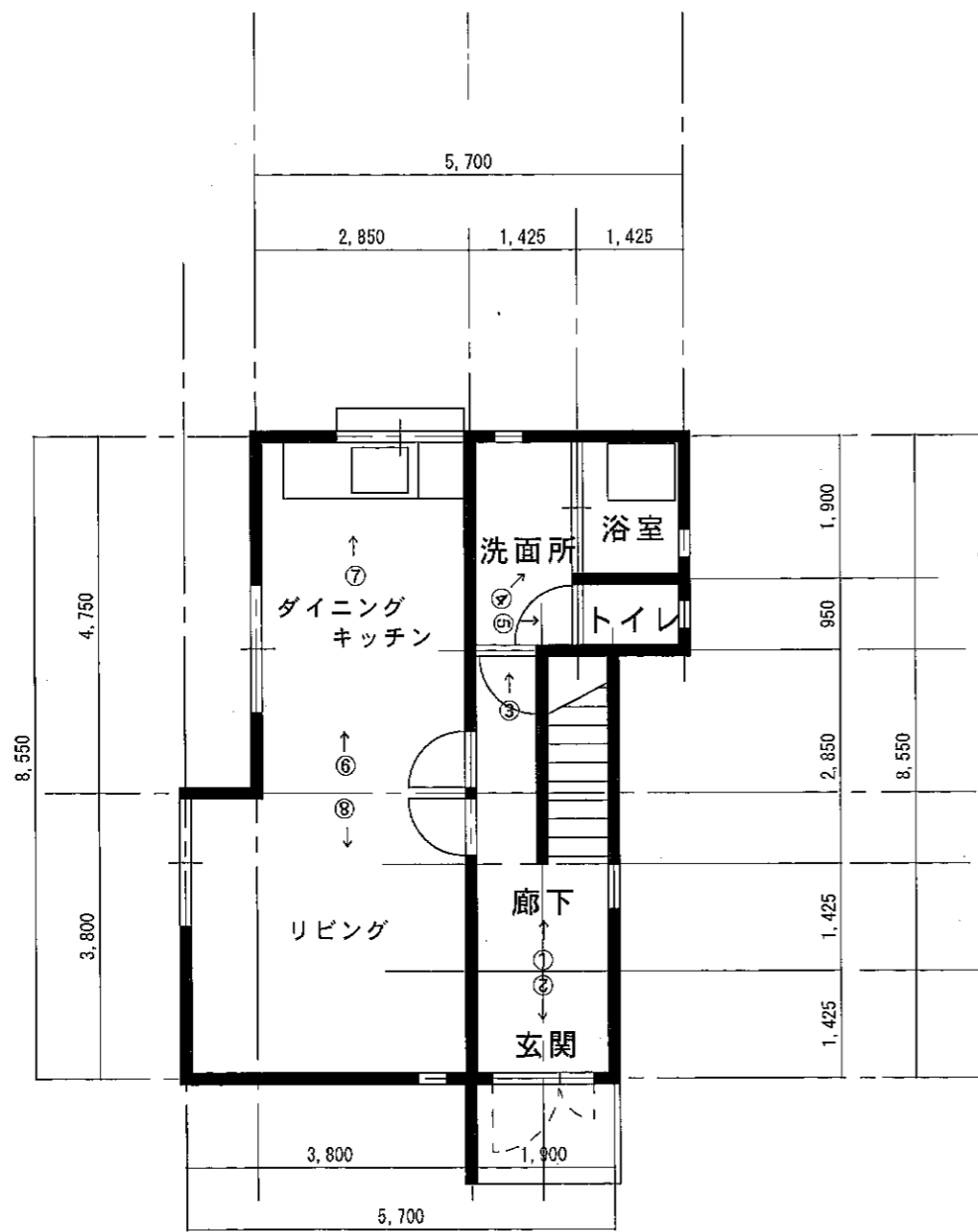
1階平面図
