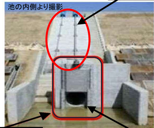
土砂吐ゲート (底樋管からの排水時に使う)
