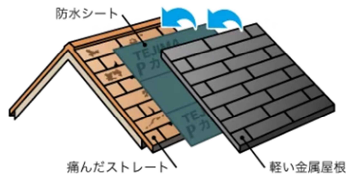
屋根及びとい改修工事 (カバー工法)
